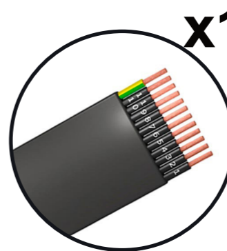
PENDENTIF (Si porte cabine) PR003249
