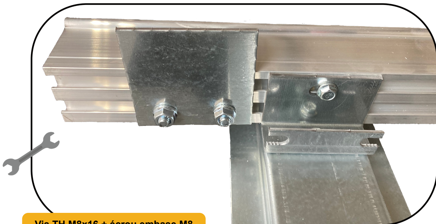
Vis TH M8x16 + écrou embase M8
